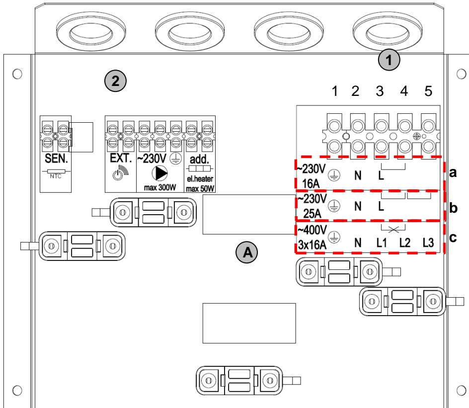
Abbildung 14: Elektrische Anschlüsse
